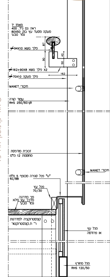
חתך 4 קני"מ 50
