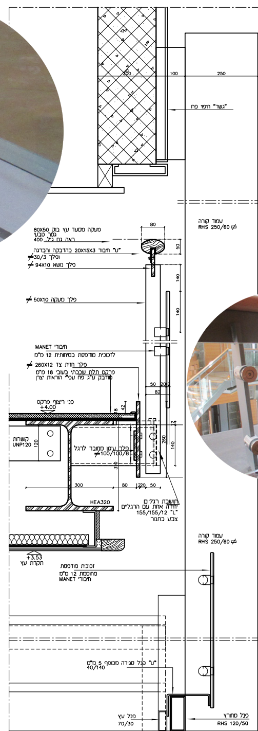
חתך 3 קני"מ 50 © אודי קרמסקי אדריכל
