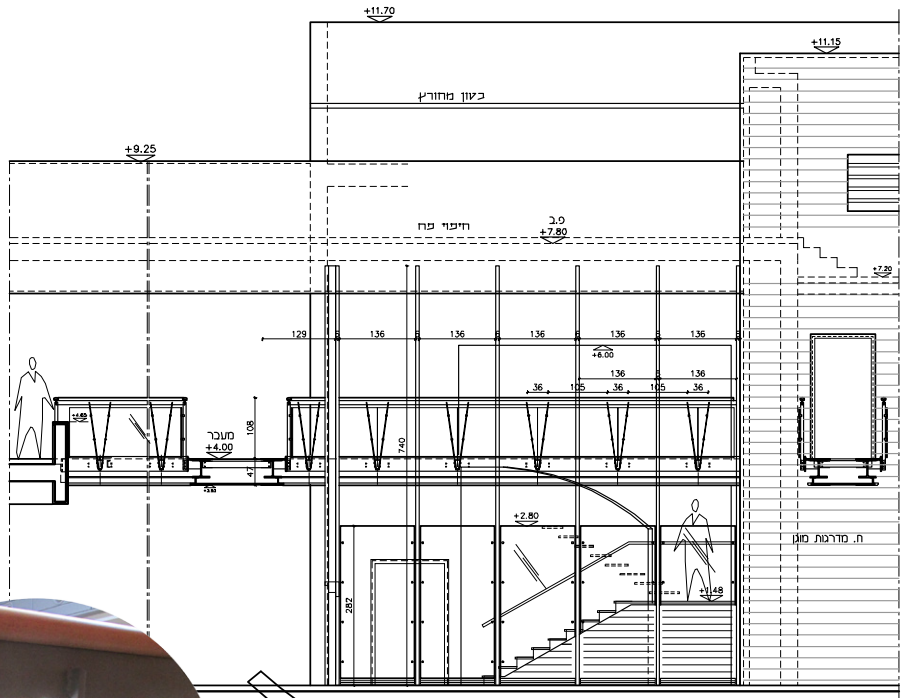
חתך 1 קני"מ 50
