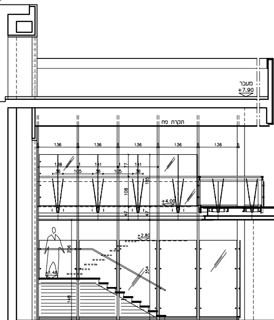
חתך 5 קני"מ 50 © אודי קרמסקי אדריכל
