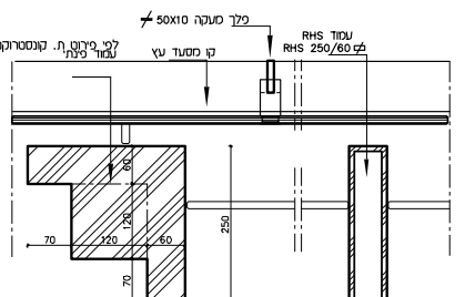
תכנית בהפלים במפלס +4.00 קני"מ 50
