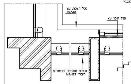
קטע תכנית בהפלים במפלס +0.00 קני"מ 50
