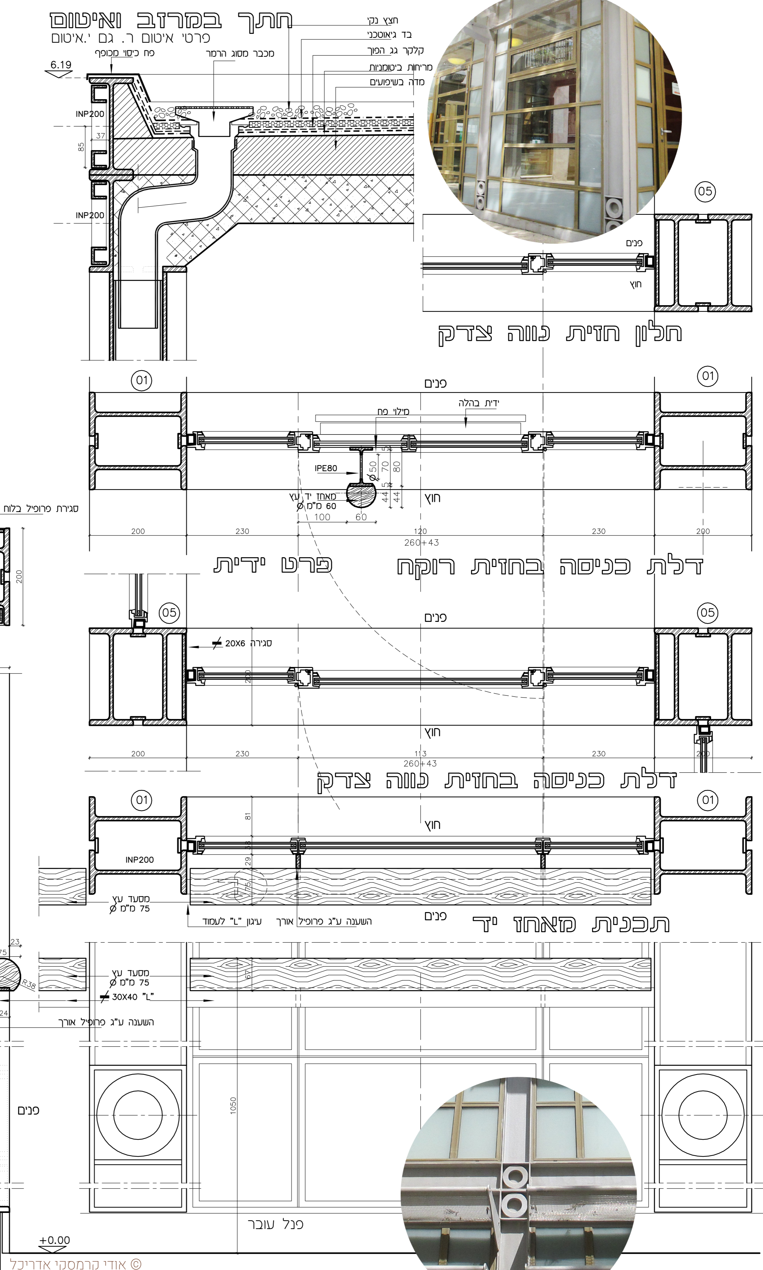
דלת וידית | חתיך קיר מסך | דלת וקבוע | חתיך בחלון | פרט איטום לכיכר | חתיך מאחז יד | חזית מאחז יד ע"ג ויטרינה | חתיך במרזב איטום
