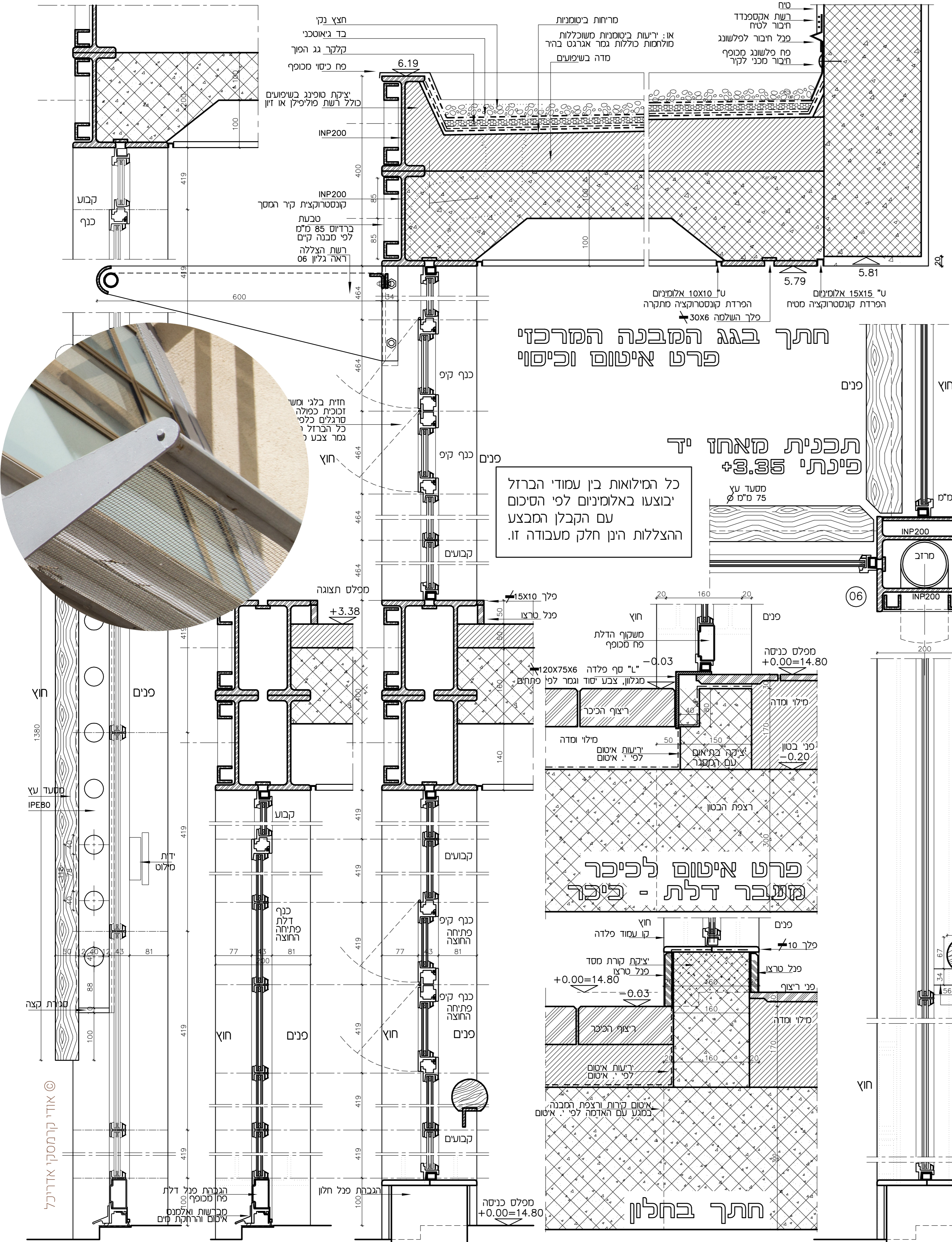
דלת וידית | חתיך קיר מסך | דלת וקבוע | חתיך בחלון | פרט איטום לכיכר | חתיך מאחז יד | חזית מאחז יד ע"ג ויטרינה | חתיך במרזב איטום
