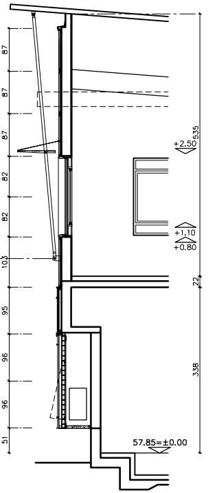
חתך בחזית מערבית קנ"מ 5:1
