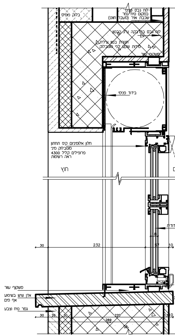
חתך אורך בחלון מונטבלוק
